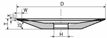
12R4 D*W*X*T*H
