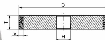
1A1 D*T*X*H
