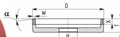
6A2 D*W*X*T*H*α°
