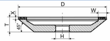
12A2-45° D*W*X*T*H
