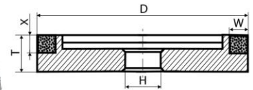
6A9 D*W*X*T*H
