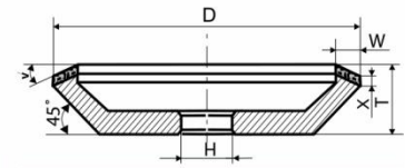
12V5-45° D*T*W*X*V*H
